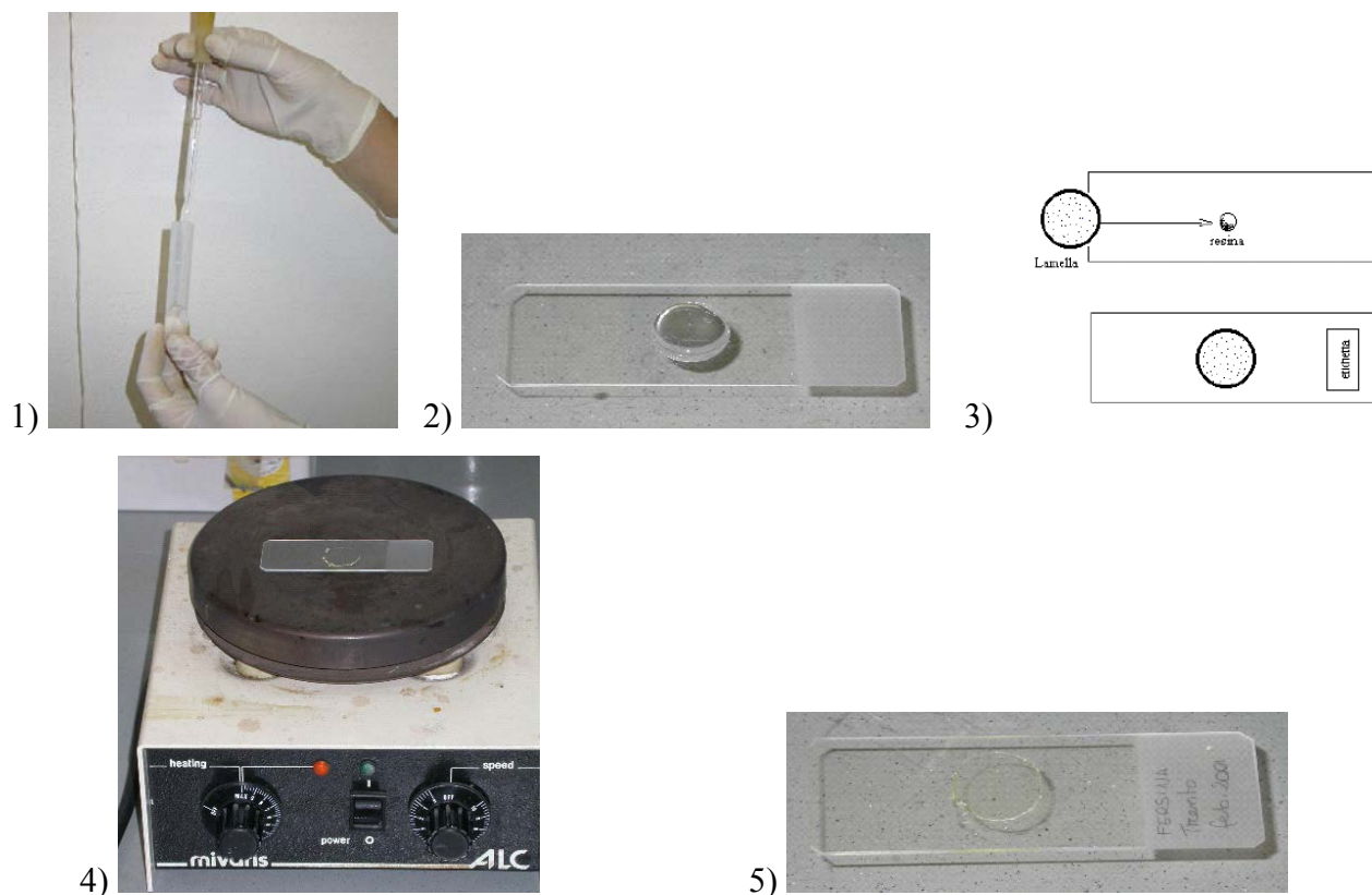
Figura 5 - Diversi passaggi durante la preparazione dei vetrini permanenti: 1) preparazione della diluizione idonea; 2) collocazione della goccia di campione (appositamente diluito) sul vetrino coprioggetto; 3) il copri oggetto dopo essiccazione viene posto sulla resina; 4) il vetrino allestito viene posto sulla piastra per far evaporare il solvente della resina; 5) il vetrino è pronto.
