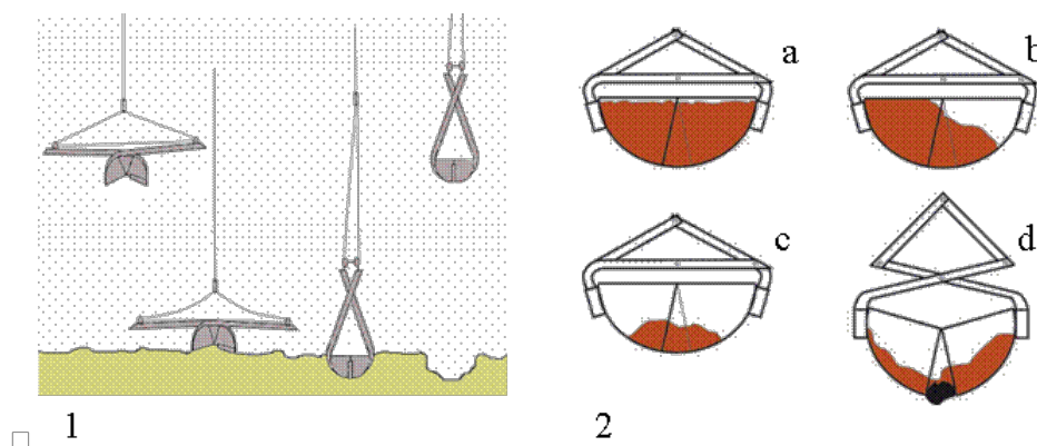
Figura 4 – (1) Schema di funzionamento e (2) raccolta di un campione da draga: a) draga con campione integro accettabile; b) campione inaccettabile dovuto ad inclinazione della draga al momento della raccolta; c) campione inaccettabile per mancato sprofondamento nel sedimento; d) campione inaccettabile per inceppamento delle ganasce con pietre.
