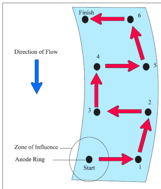
Figura 1 - Schema campionamento
