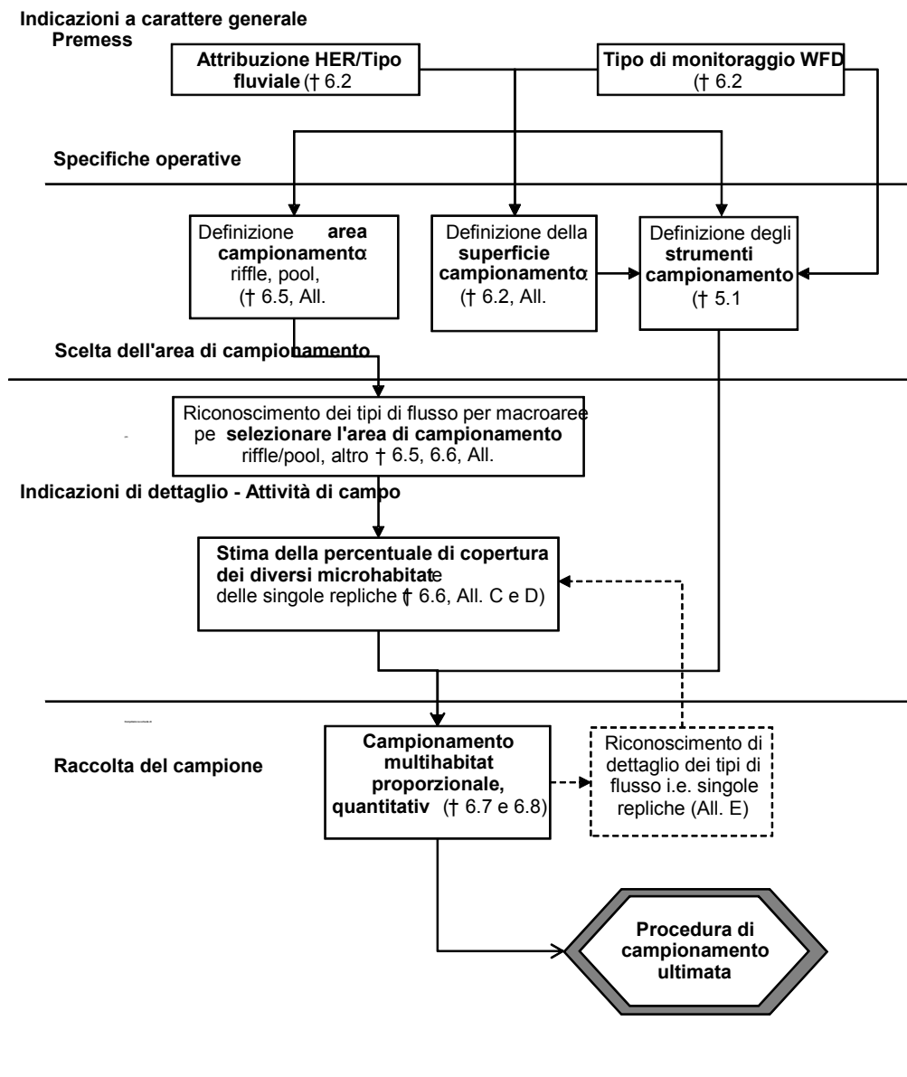
Figura 3 - Diagramma illustrante i principali passaggi della procedura di campionamento (modificato da [6]).
